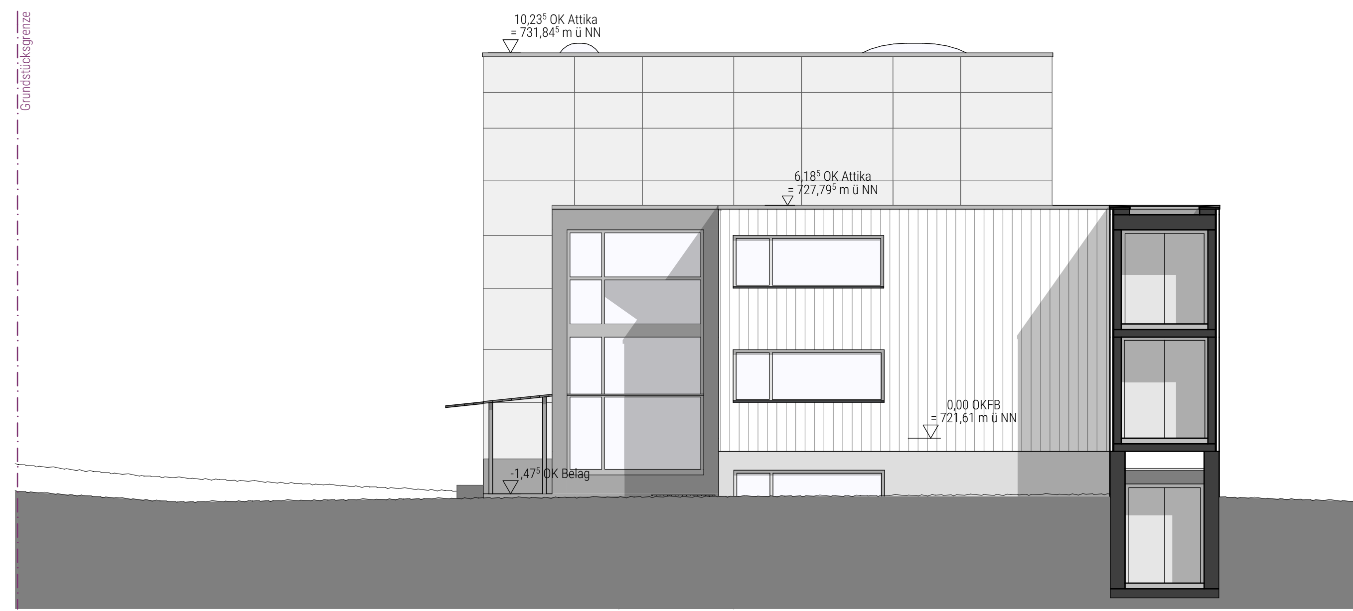
Ansicht Süd M 1:100
