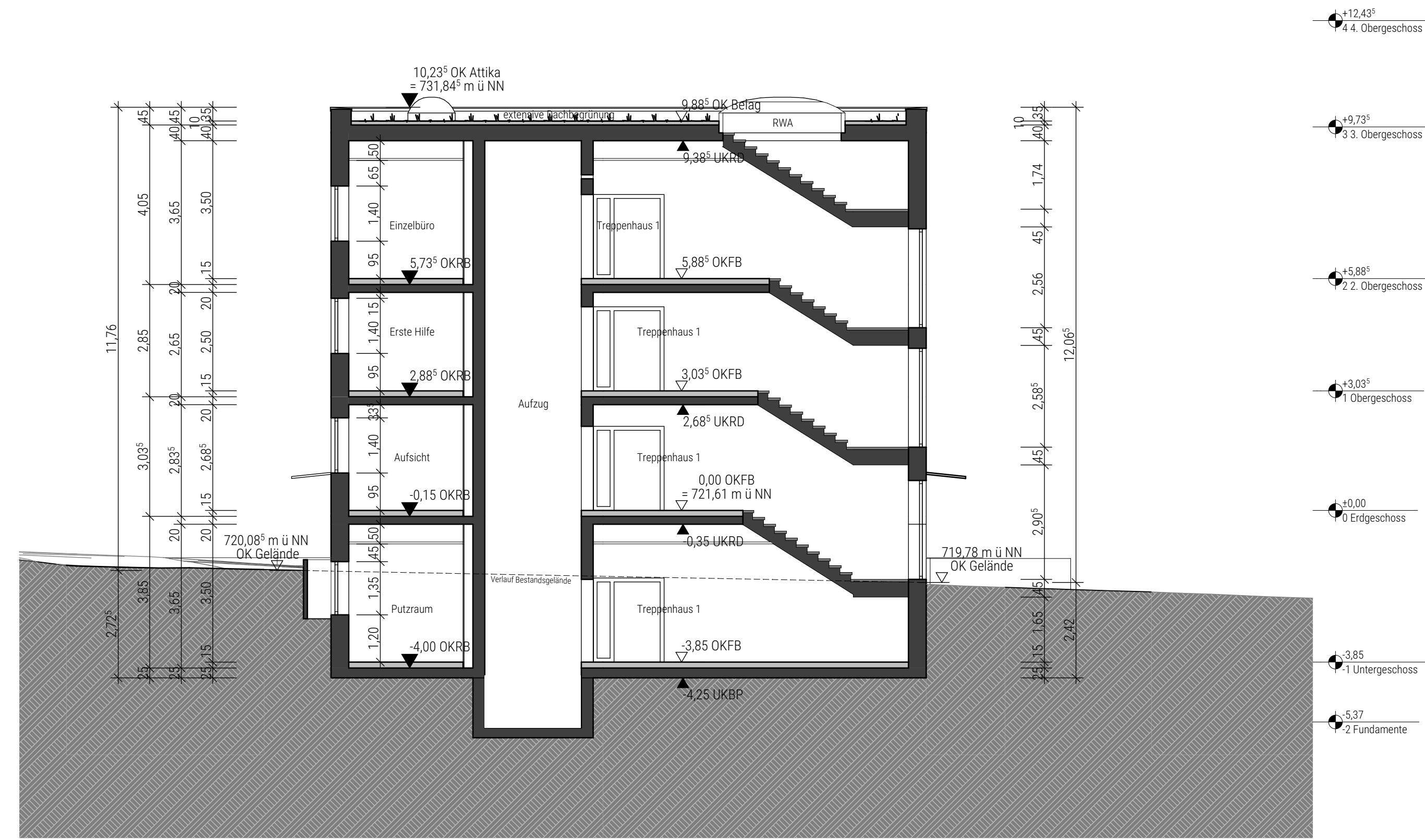
Schnitt A - A M 1:100
