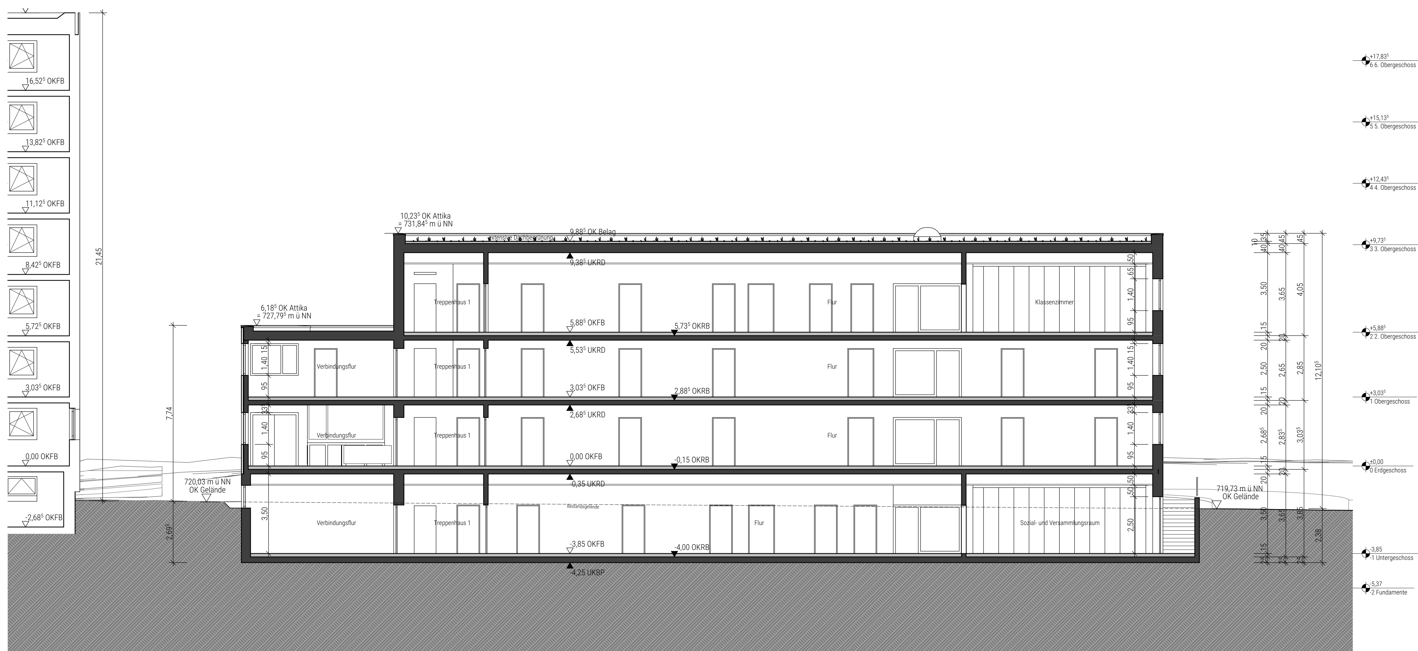
Schnitt D - D M 1:100
