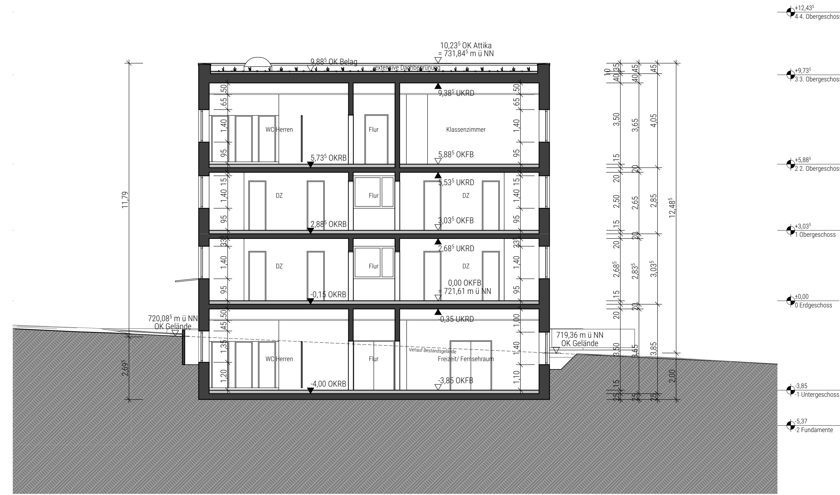
Schnitt B - B M 1:100
